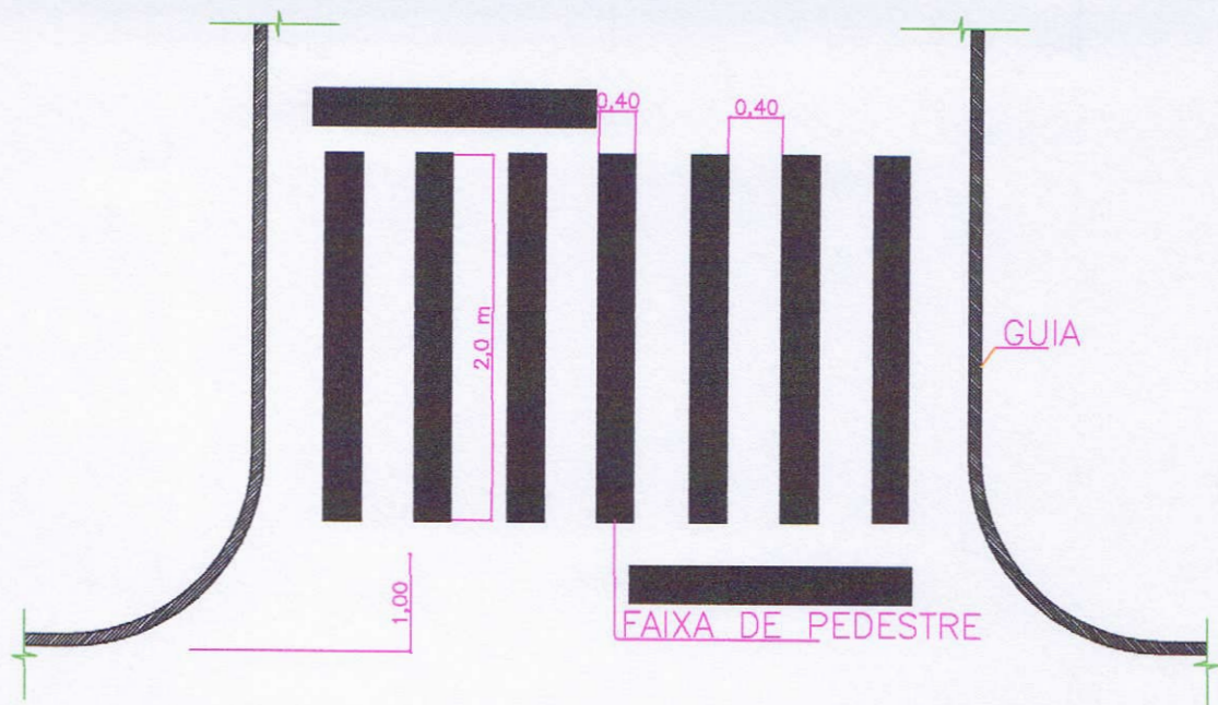
DETALHE DE FAIXA DE PEDESTRE ZEBRADA
