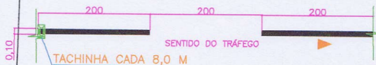
DETALHE DE LINHA TRACEJADA E TACHAS
