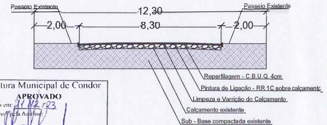
PERFIL TRANSVERSAL RUA JOSÉ FERNANDES KRUGER PAVIMENTAÇÃO C.B.U.Q - SOBRE CALÇAMENTO EXISTENTE
