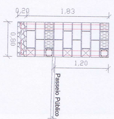
Ancoragem muro 03 Escala: 1/50
