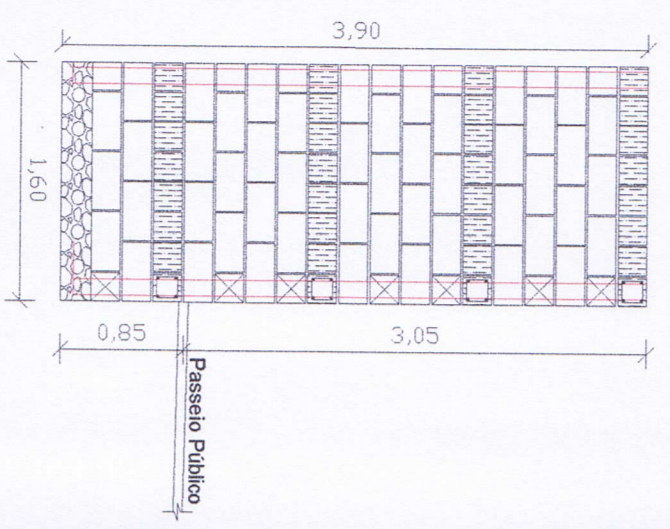
Ancoragem muro 01 Escala: 1/50
